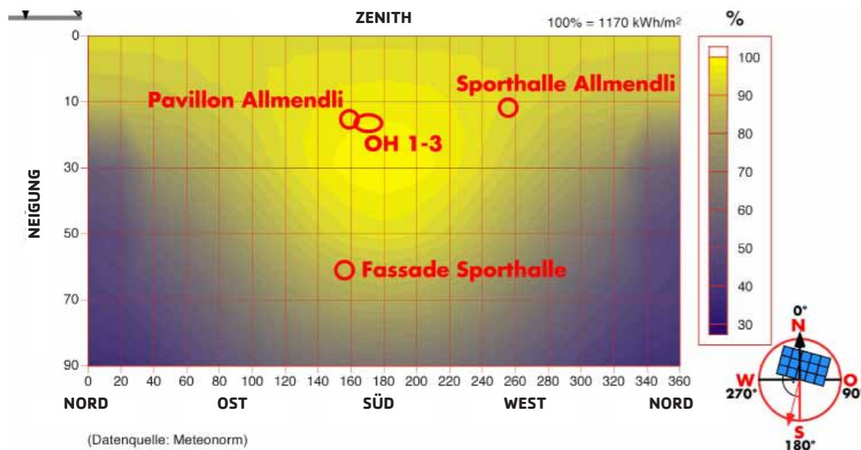
JAHRES-STRAHLUNGSANGEBOT IM RAUM ZÜRICH
